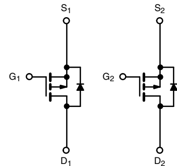
P-Channel MOSFET P-Channel MOSFET
